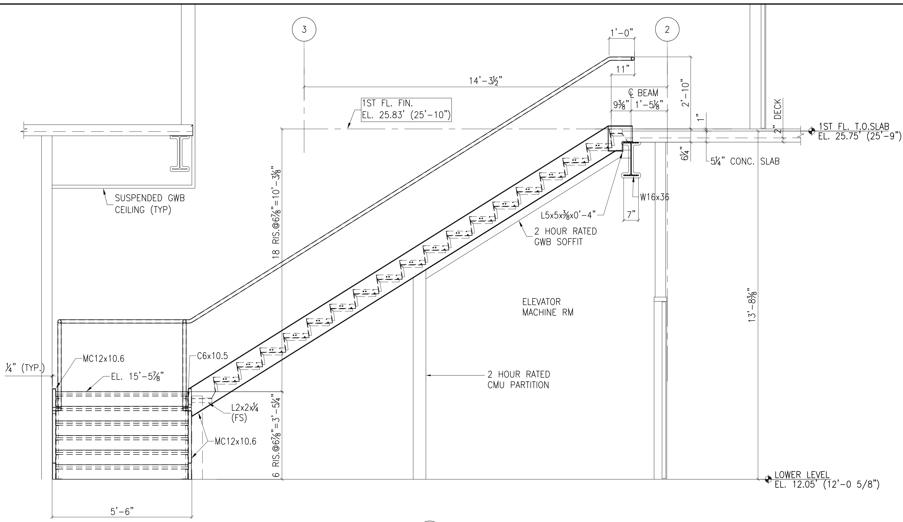
A SECTION ST8 SCALE: 1/2" = 1'-0"
