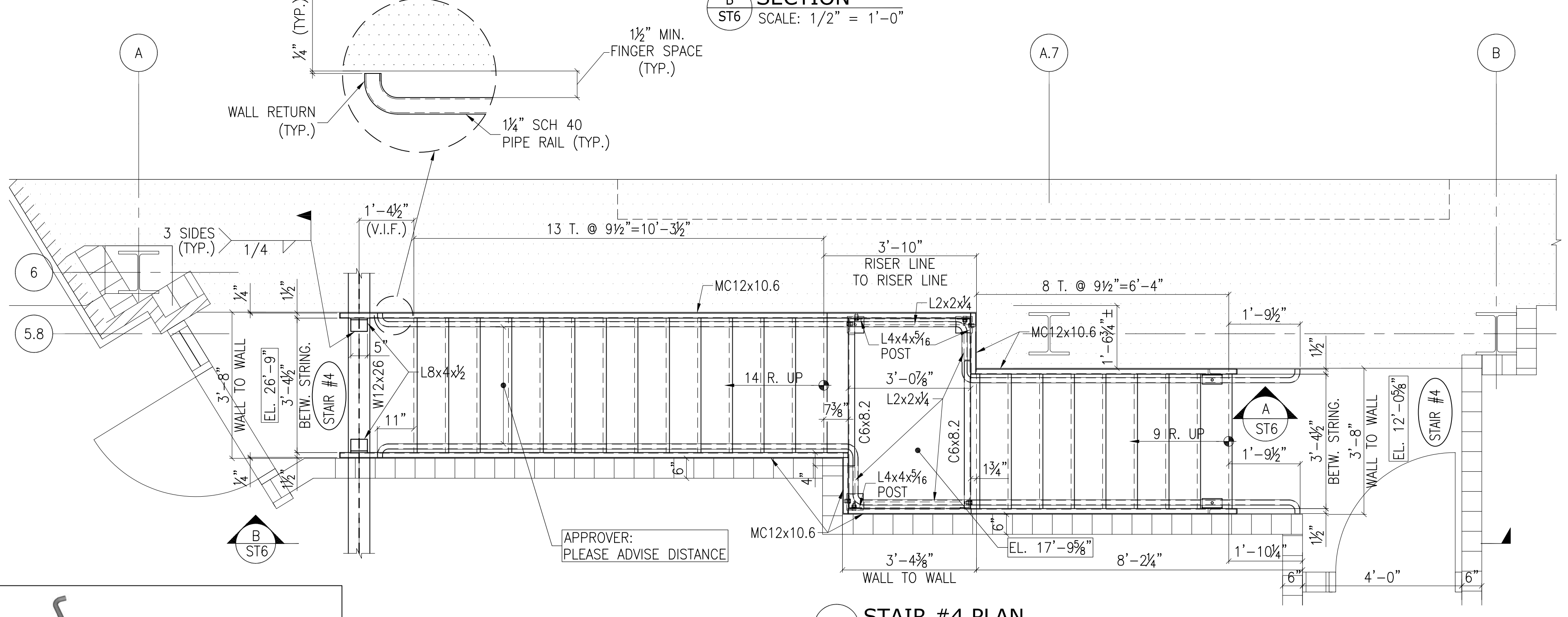
STAIR #4 PLAN ST6 SCALE: 1/2" = 1'-0"
