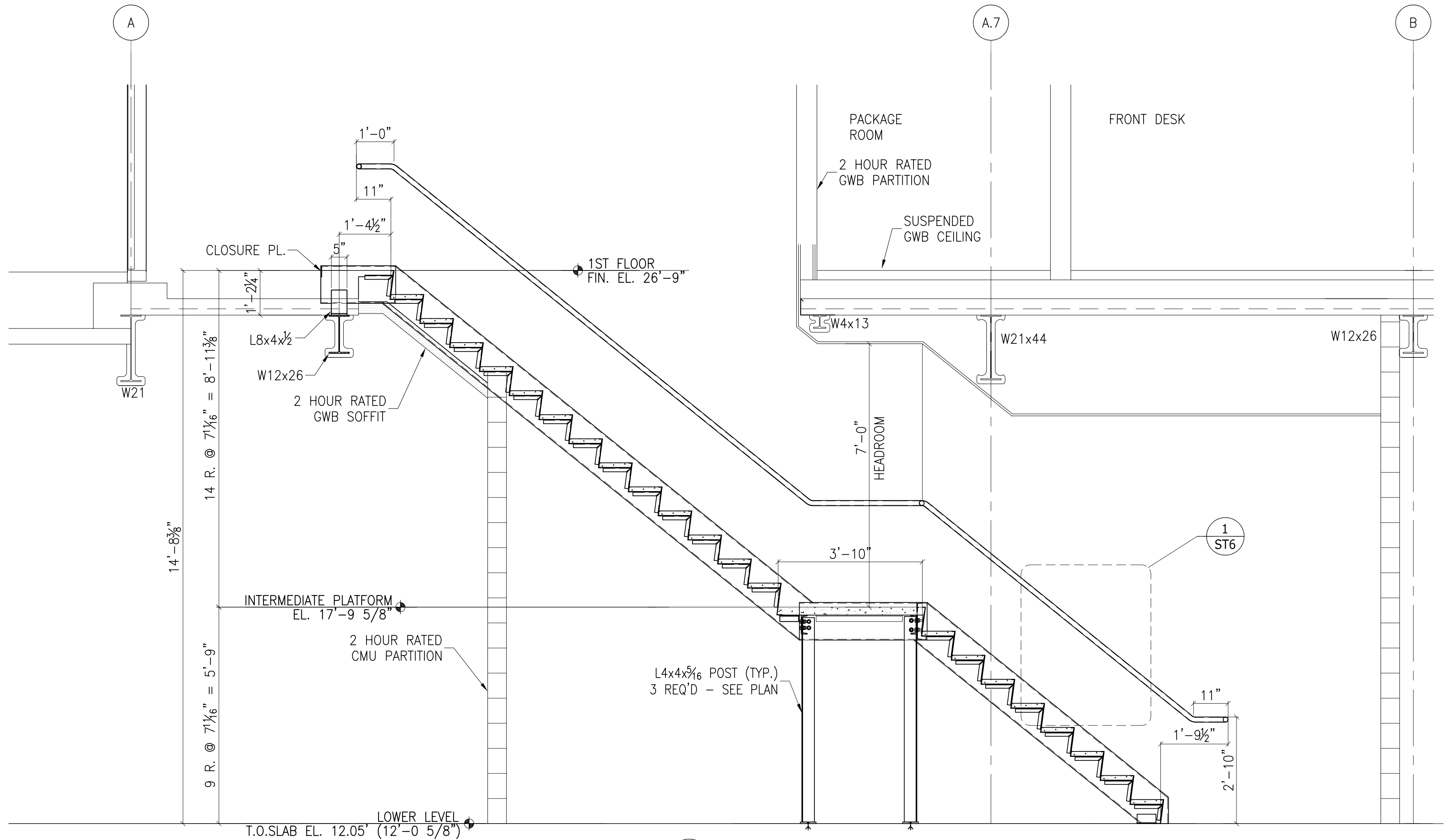
B SECTION ST6 SCALE: 1/2" = 1'-0"
